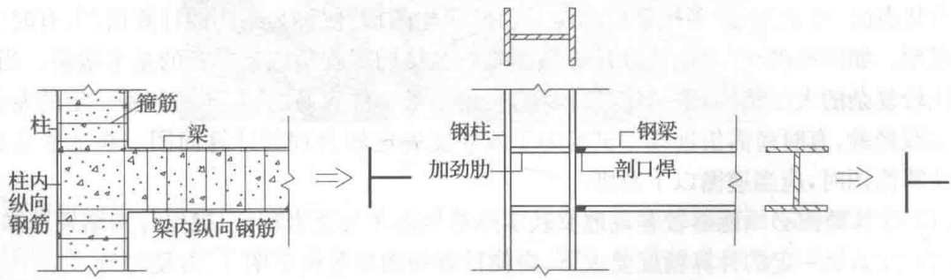
(a) 钢筋混凝土框架结点
