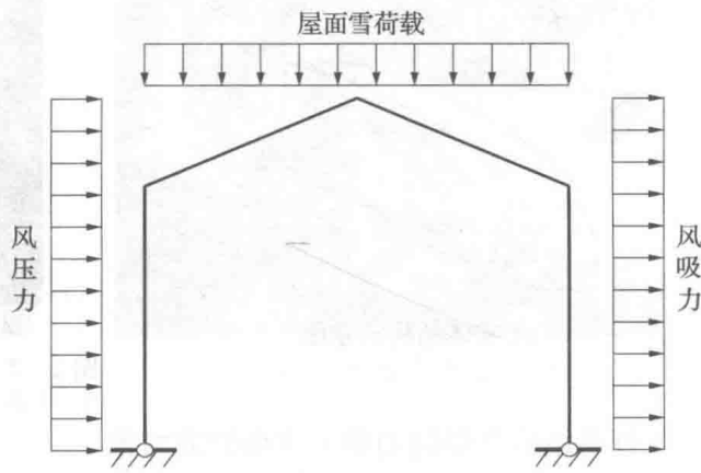
(b) 简化结构
