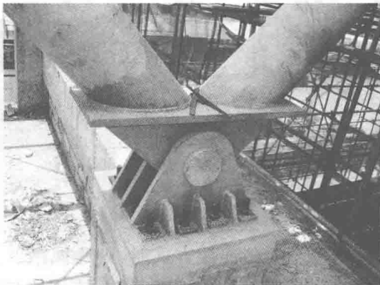
(a) 某工程的固定铰支座
