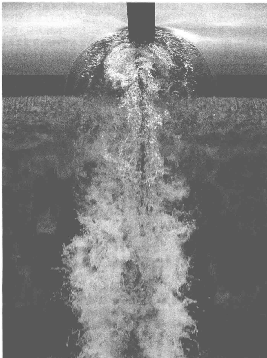
一架飞机机翼顶端产生的涡旋中的湍流
