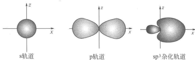
图 1-2 s 、 p 轨道和 sp^3 杂化轨道的形状
