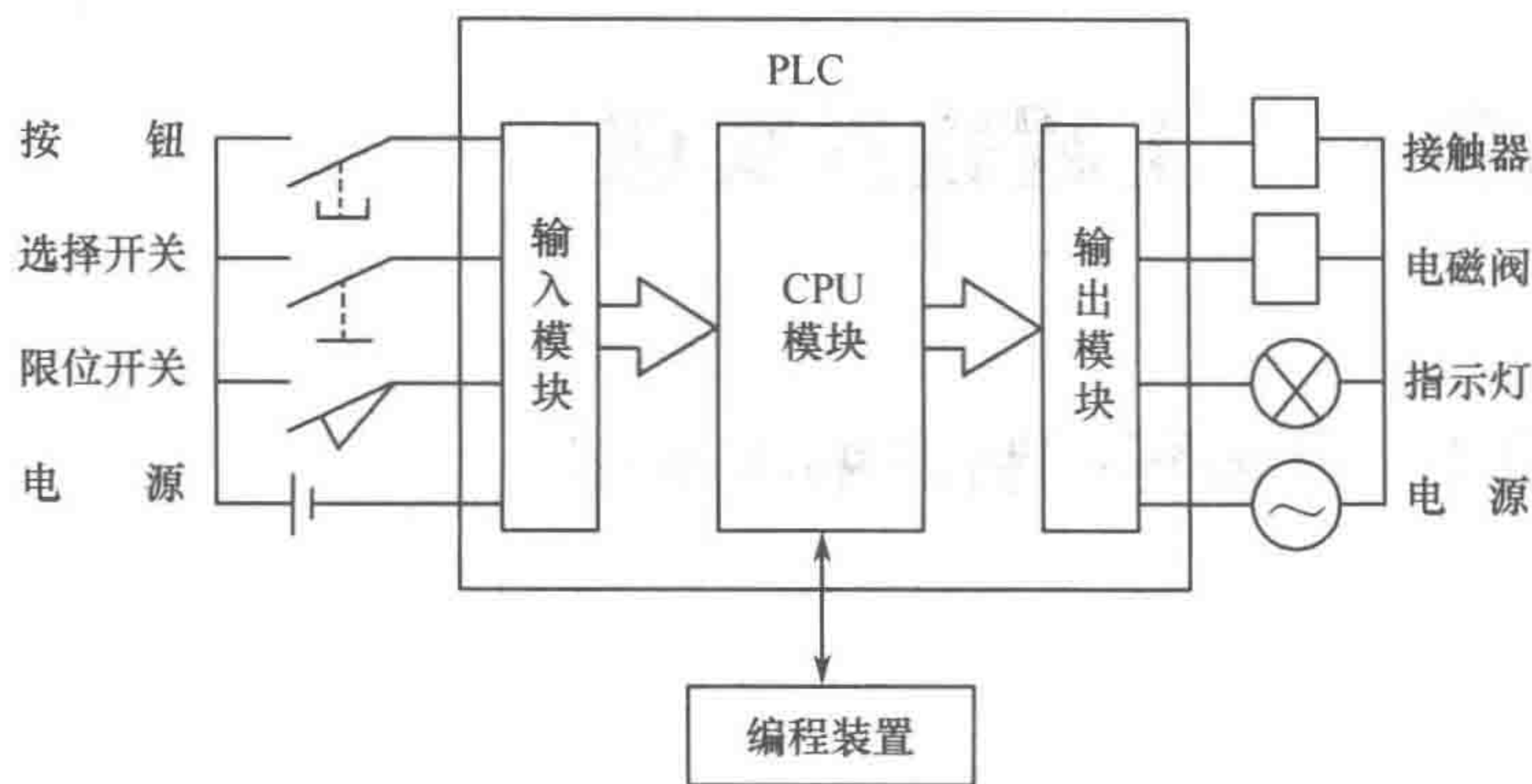
图 1-1-1 PLC 基本结构
