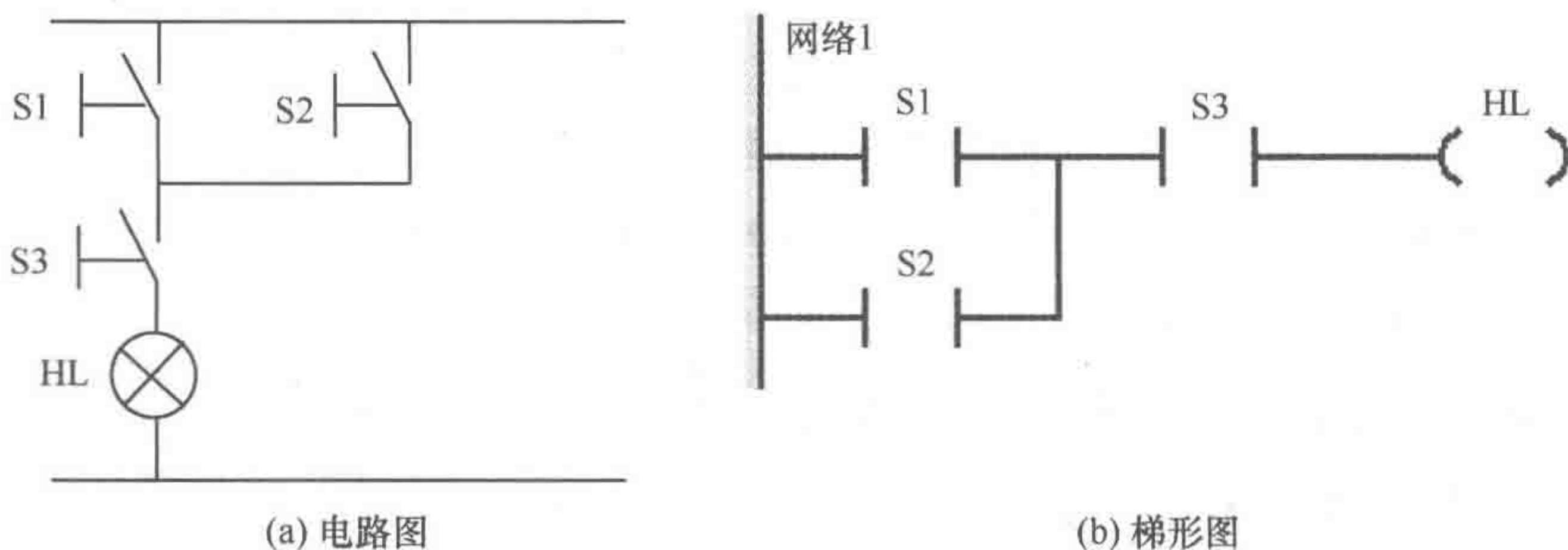
图 1-1-12 电路图与梯形图
