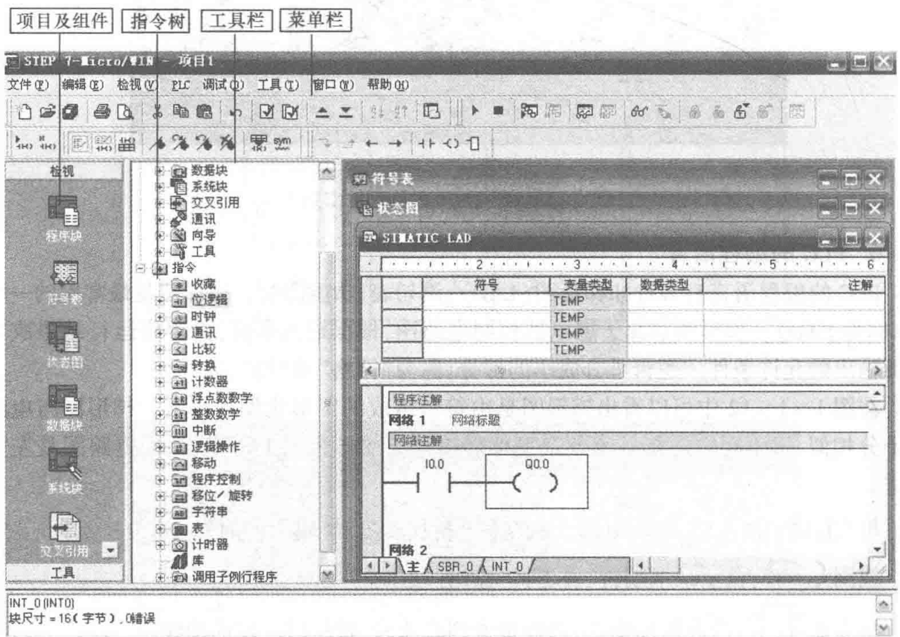
图 1 – 1 – 14 STEP7 – Micro/WIN 4.0 操作界面图
