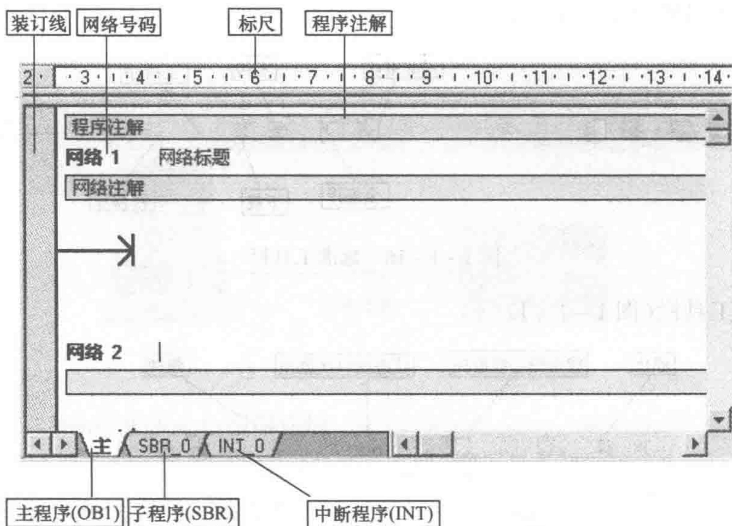
图 1-1-20 程序块编辑窗口
