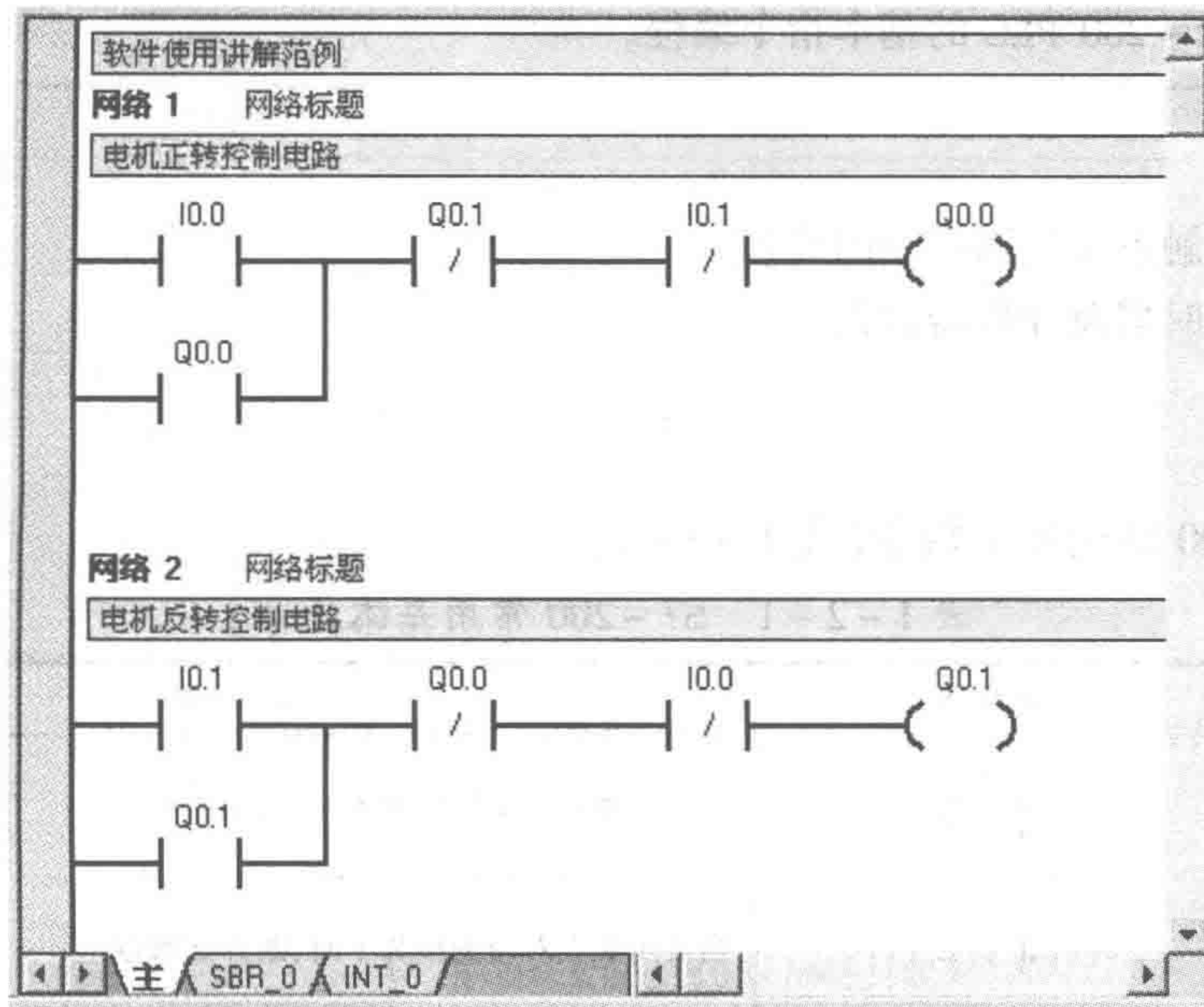
图 1-1-21 程序 1 梯形图
