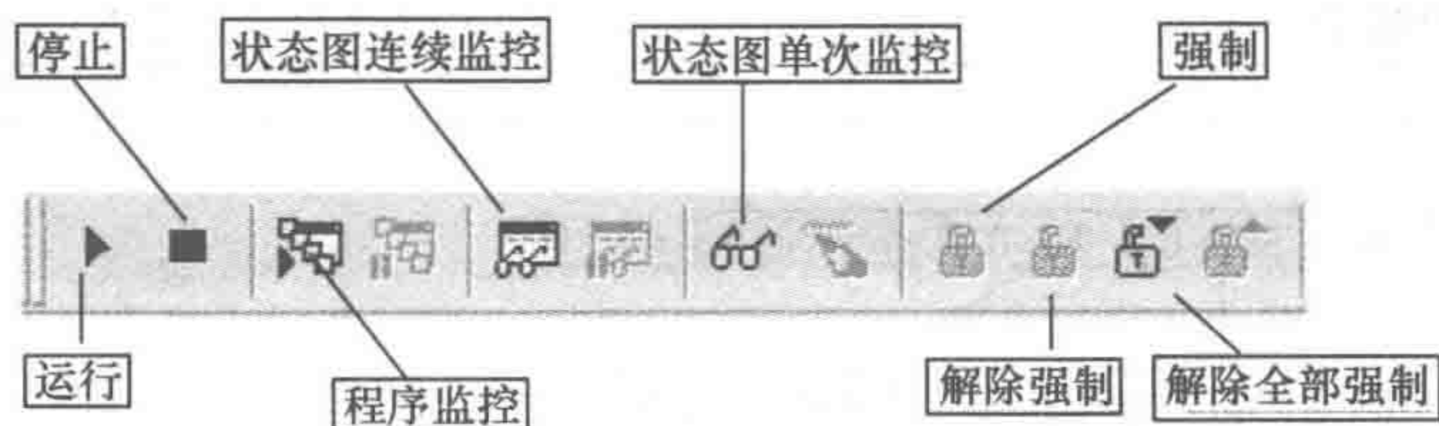
图 1-1-17 调试工具栏
