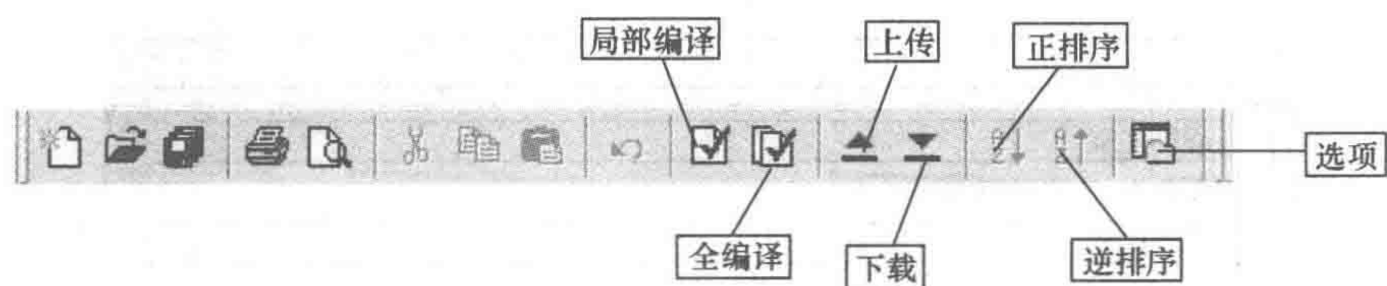
图 1-1-16 标准工具栏
