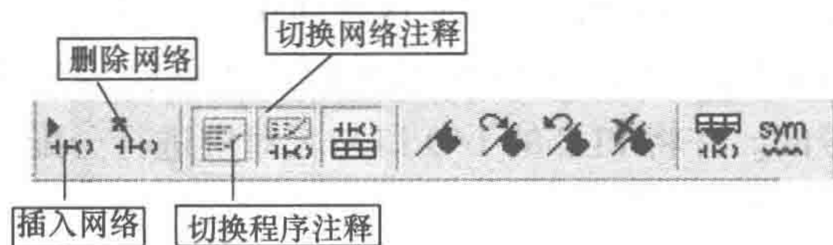
图 1-1-18 常用工具栏
