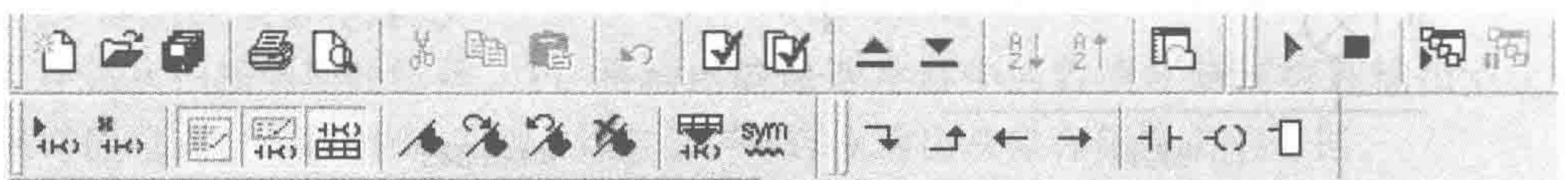
图 1 – 1 – 15 工具栏
