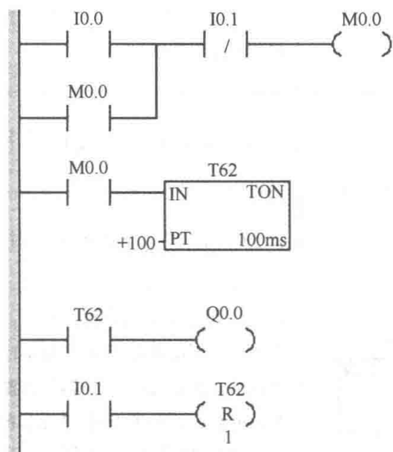
图 1-1-22 程序 2 梯形图
