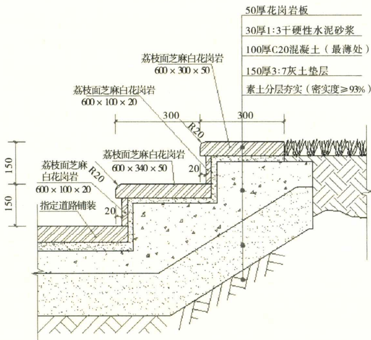
图1-3 台阶施工详图
