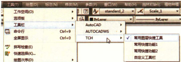
图2-4 工具栏菜单
