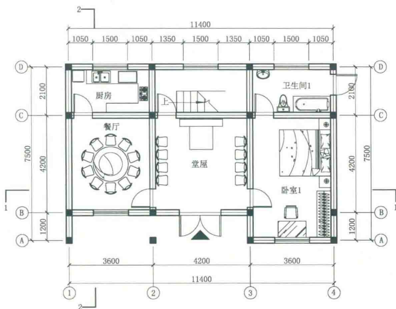
一层平面布置图
