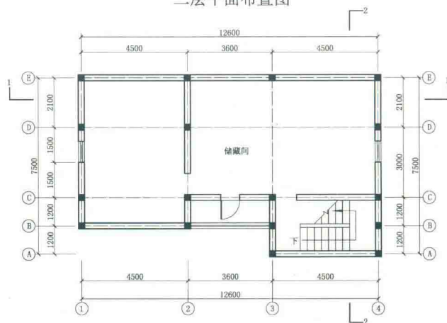
二层平面布置图
