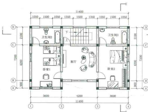
二层平面布置图
