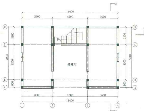
三层平面布置图
