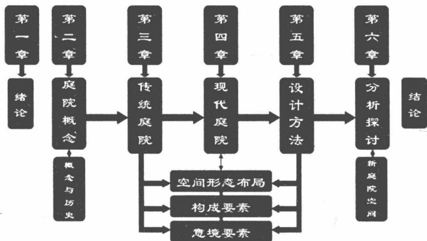
图 1-1 文章结构
