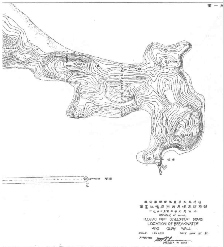
附擬築防波堤及西附岸墻位置圖
