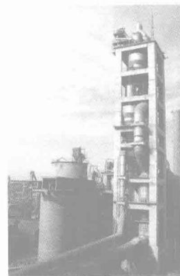
公司设计的山西中铝二水泥预分解系统 Preheating system of Wuzhong No.2 cement factory
