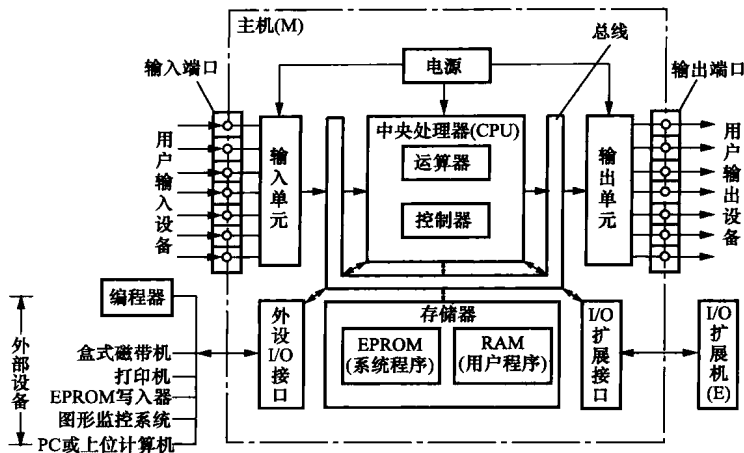
图 1-3 PLC 硬件结构简化框图
