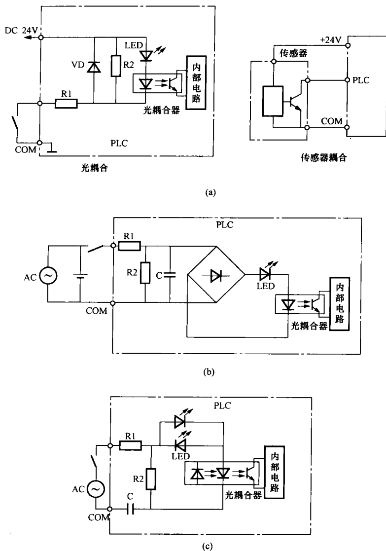
图 1-4 开关量输入接口电路
