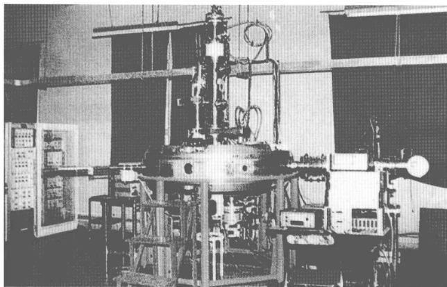
20世纪90年代国家自然科学基金会的重大项目，世界第一台“超灵敏小型回旋加速器质谱计”在中国科学院上海原子核研究所诞生
