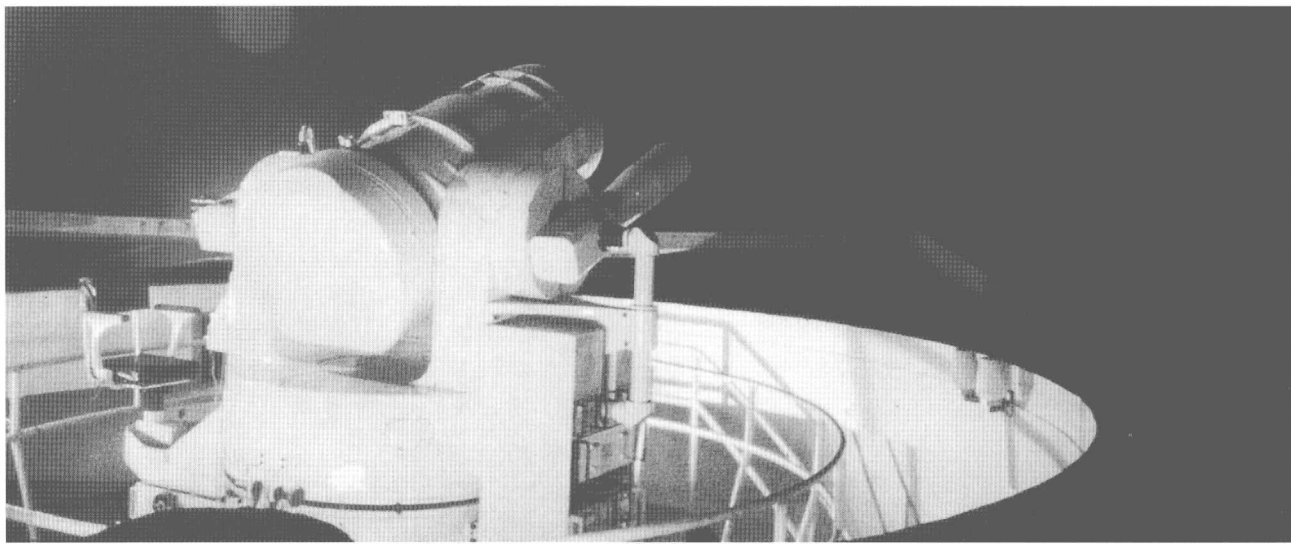
20世纪80年代中国科学院上海天文台与有关单位协作研制的60厘米人造卫星激光测距仪
