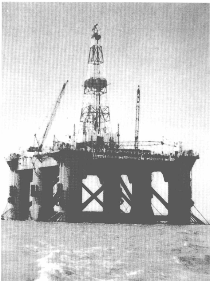
20 世纪 80 年代上海船厂自行设计建造的中国第一艘半潜式平台，采用独创的水上合龙、浮力顶升等先进工艺
