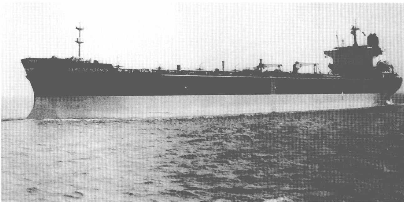
20 世纪 90 年代上海沪东造船厂建造的 68600 吨油轮，能装载两种闪点 60^{\circ}\text{C} 以下的原油，入 ZC 无限航区
