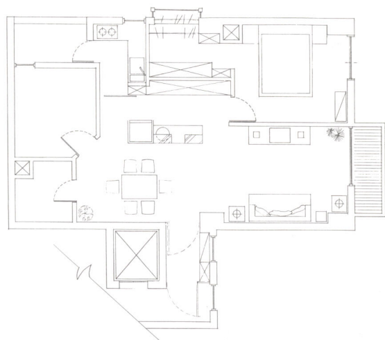
平面配置图
