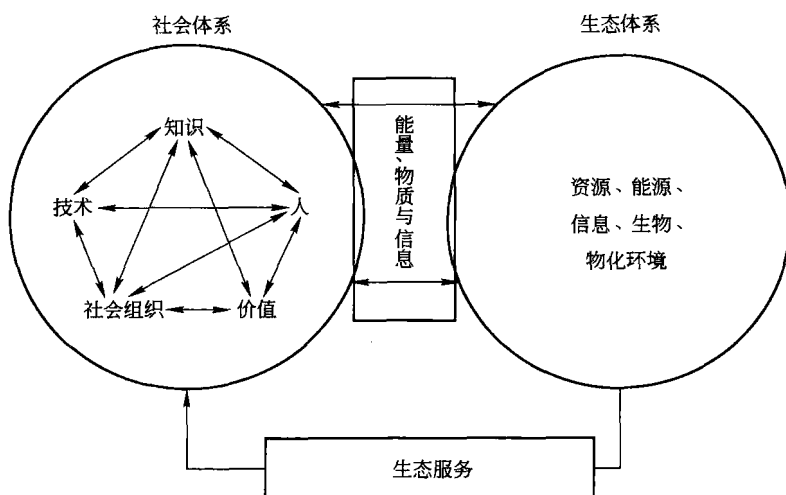
图 1-2 生态与社会体系间的能量与物质流动
