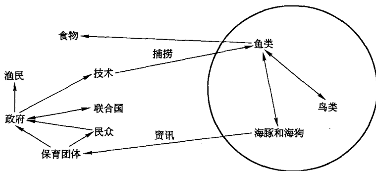
图 1-3 生态与社会体系间的链效应（海洋商业捕鱼效应）
