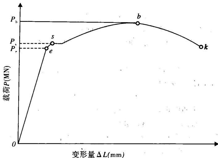
图 1-3-2 低碳钢的拉伸曲线
