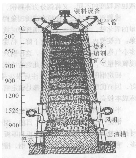
图 1-1-1 炼铁高炉的示意图
