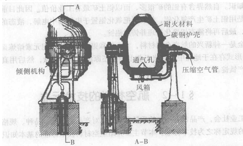
图 1-1-2 炼钢转炉示意图
