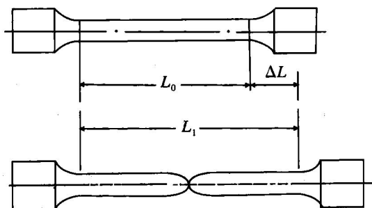
图 1-3-3 拉伸试样断裂前后的标距
