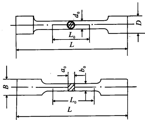
图 1-3-1 标准拉伸试样
