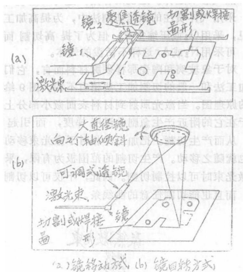
图5.激光束的偏向方法
