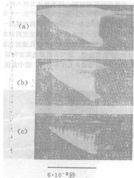
图5. 产生于不同平均激光强度 \bar{I}_L 的三张打孔过程的条纹照片: (a) 5 \times 10^7 瓦/厘米 2 ; (b) 3 \times 10^7 瓦/厘米 2 ; (c) 1.7 \times 10^7 瓦/厘米 2 , 激光脉 1.5 \times 10^{-6} 秒。
