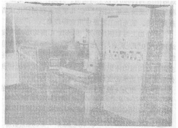
图3. 红宝石激光加工机 (日本东芝公司制LAR-502型)
