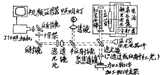
图4. 红宝石激光器加工机的结构
