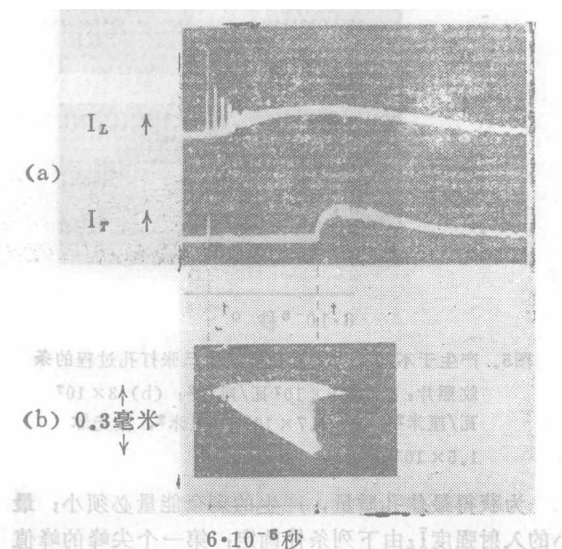
图2. (a) 入射光和透射光的时间特性, (b) 由条纹照相相机摄取的打孔过程的相片。激光束从上面会聚在0.3毫米厚的靶上。
