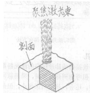
图9.激光切割
