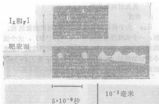
图3. 扩展时标的示波器照片和条纹照片。
