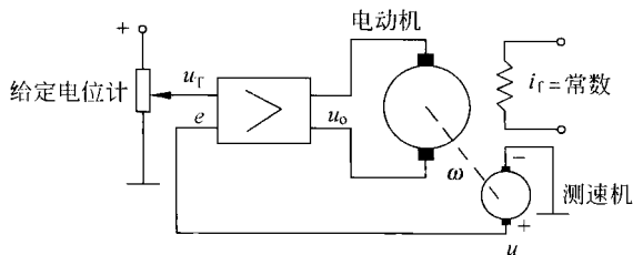
图 1-6 闭环调速系统原理图
