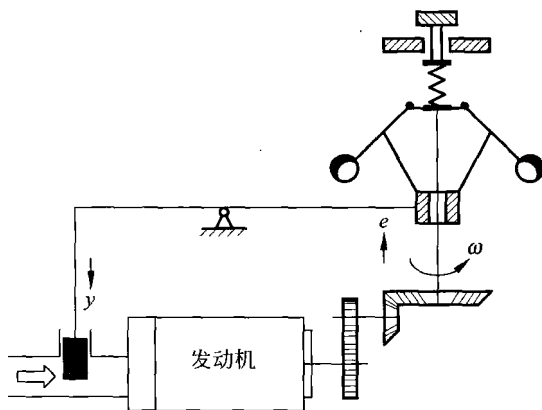
图 1-8 离心调速器
