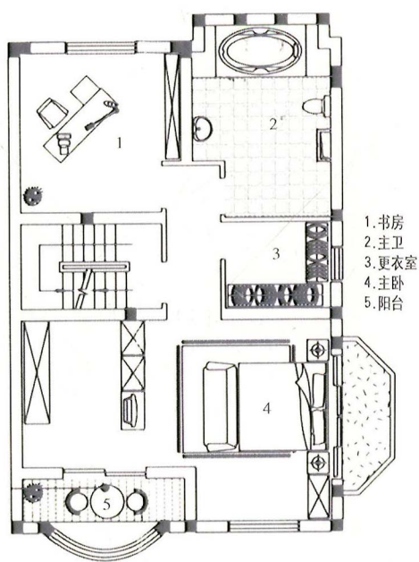
平面图
