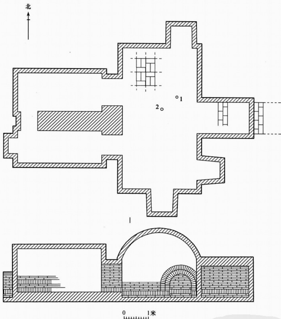
图二 独家墩墓墓葬形制
