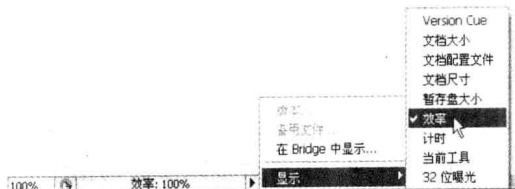
图 1-25 状态栏菜单
