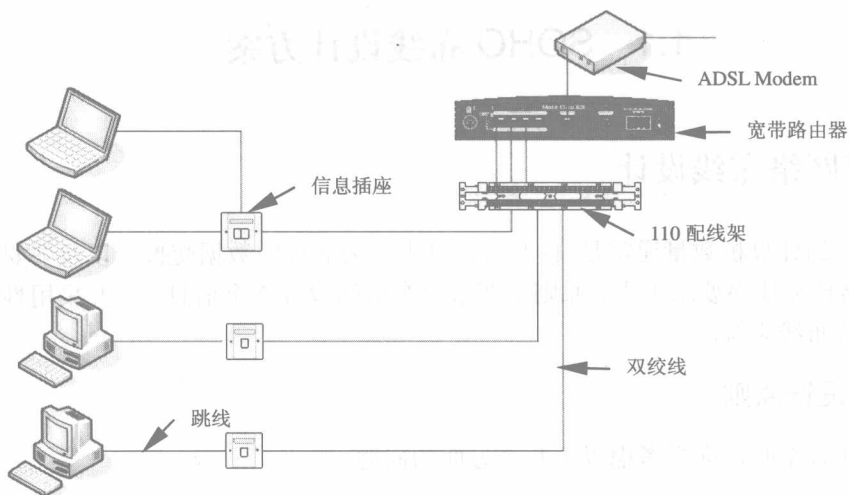
图 1-2 110 配线架方案
