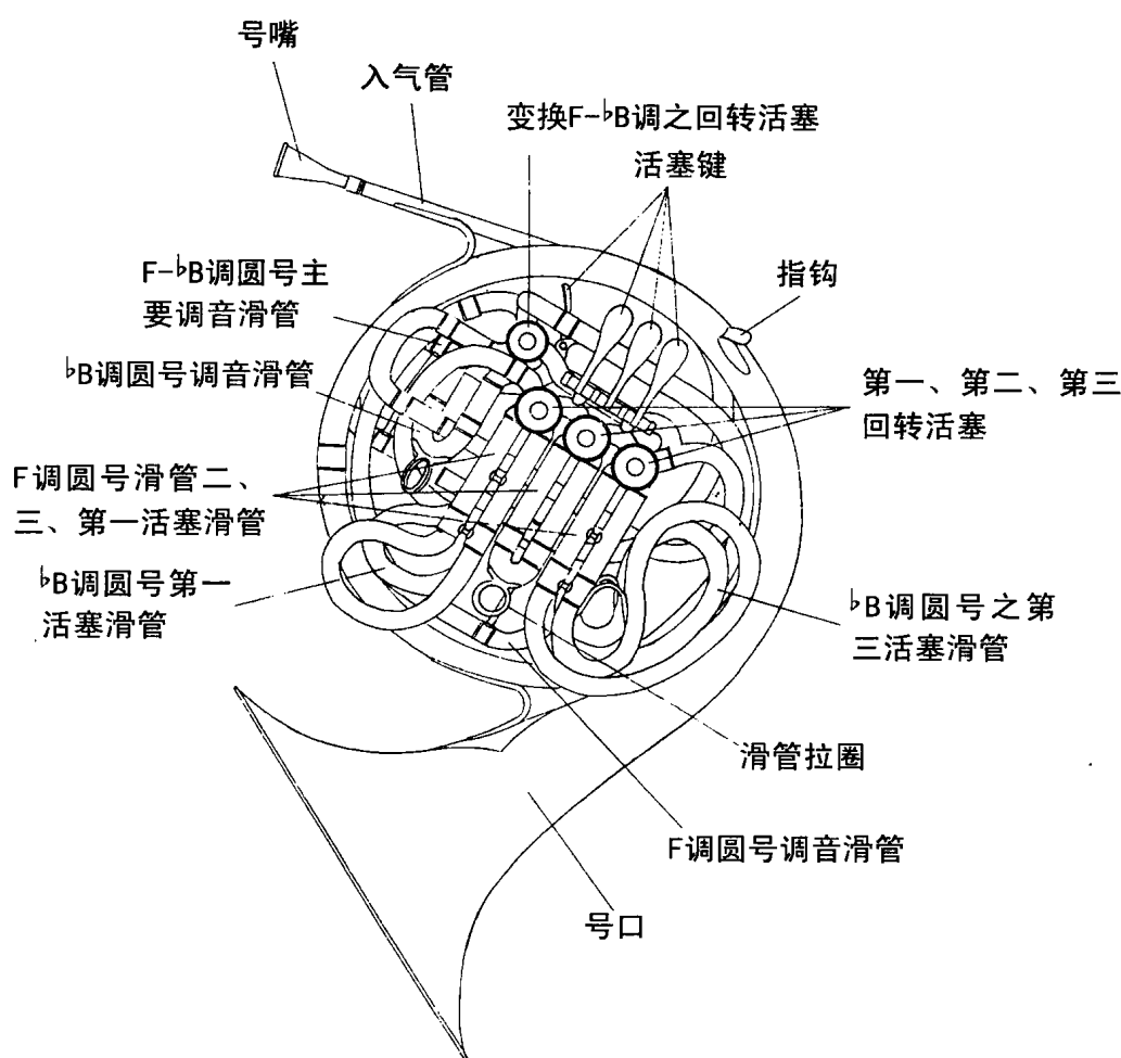
圆号的各部件
