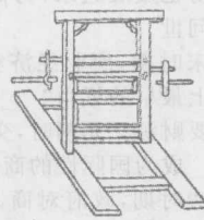
图二 元代木棉搅车
