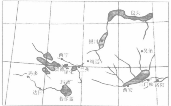
距今340万~170万年 前黄河水系格局
