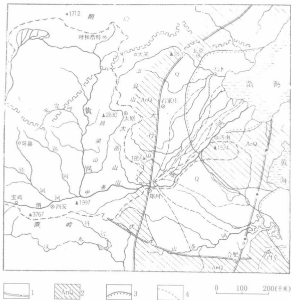
黄河古河道展布及全新世海侵(渤海)最大范围略图
