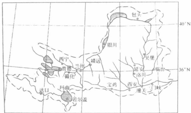
距今 110 万~14 万年前黄河中上游水系格局
