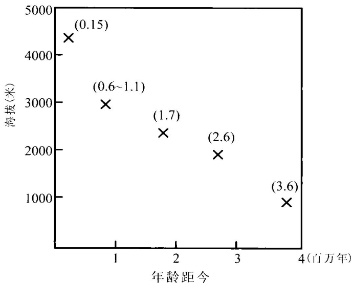
最近400多万年以来 青藏高原隆升过程示 意图
