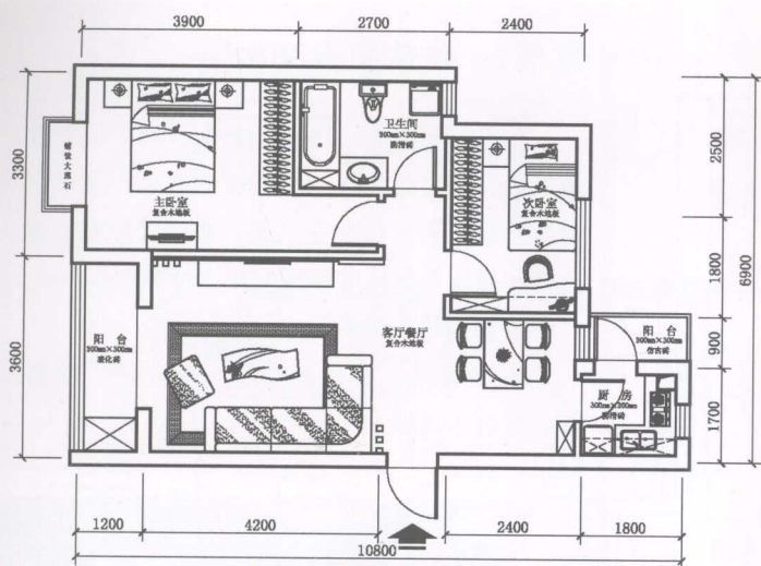
▲ 平面布置图
