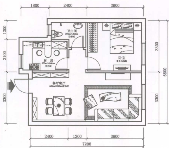
▲ 平面布置图
