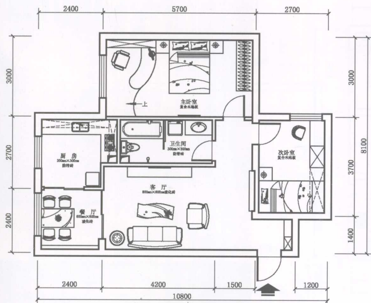
▲ 平面布置图
