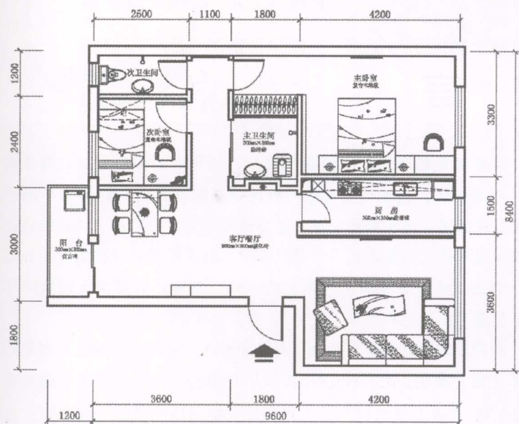
▲ 平面布置图
