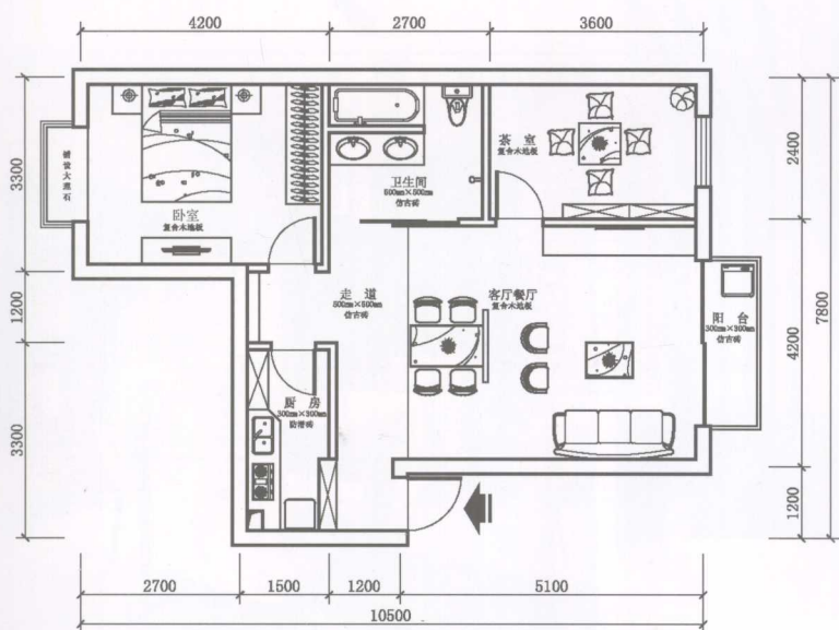
▲ 平面布置图
