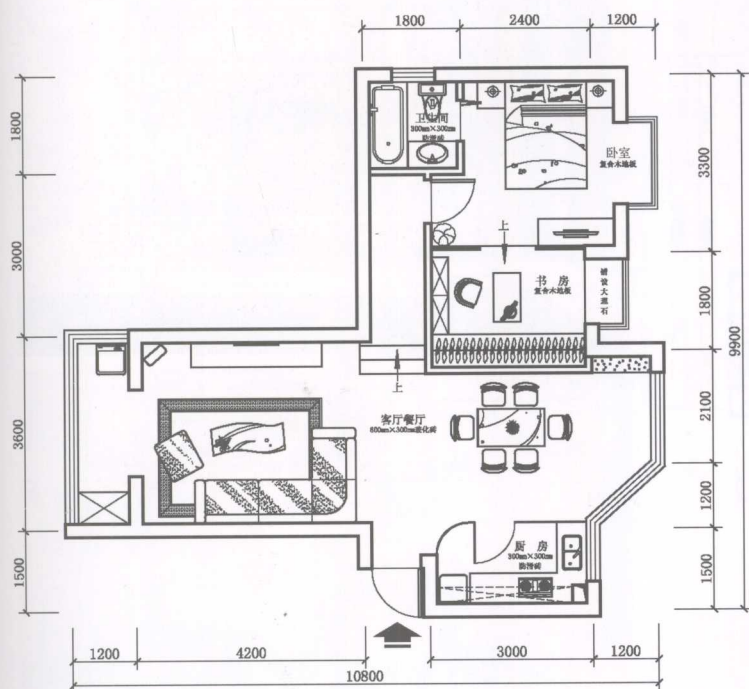
▲ 平面布置图
