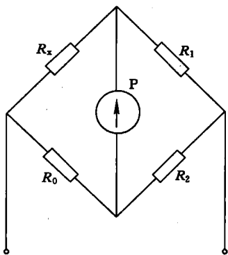
图 1-1 零值法测电阻
