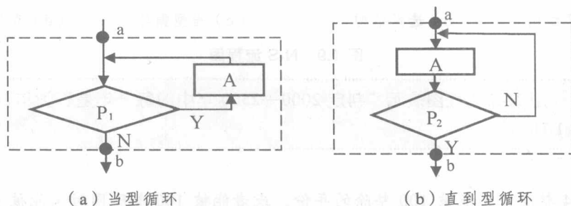
图 1.7 循环结构
