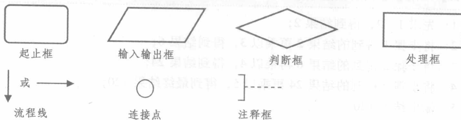
图 1.3 流程图符号
