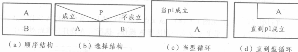
图 1.9 N-S 流程图
