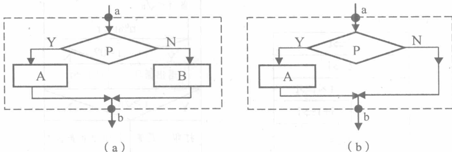
图 1.6 选择结构
