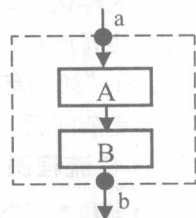
图 1.5 顺序结构
