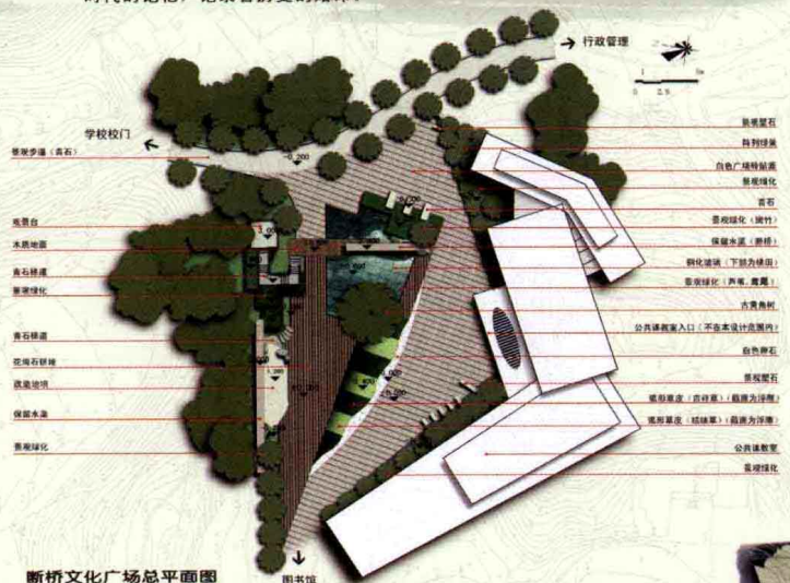
断桥文化广场总平面图
