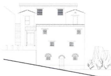
南立面图
