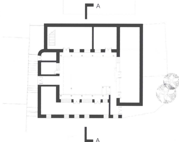
一层平面图
