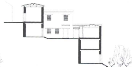
B-B剖面图
