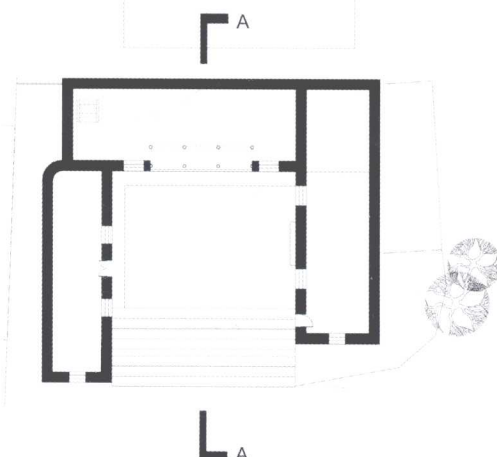
二层平面图
