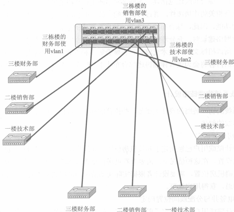
图 1-5 详细拓扑图
