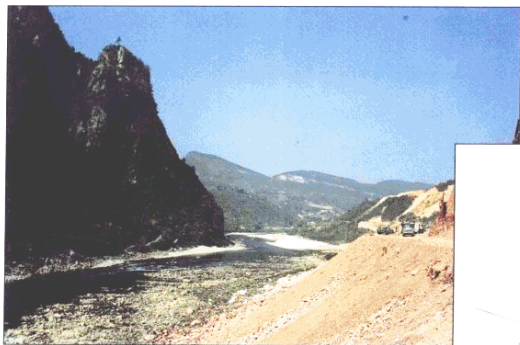
大庸魚潭電站位於永定區溫塘鎮仙街河，蓄水位250米，壩高56.5米，庫容1.315億立方米，裝機5萬千瓦，年發電量5.3億度，預計1994年竣工。圖為施工現場。
