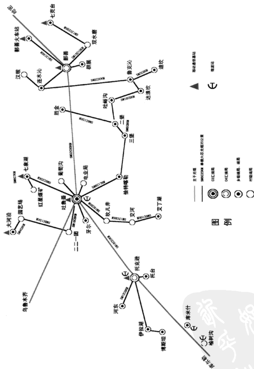
1998年吐鲁番地区电信电路示意图
