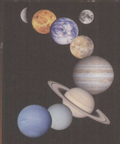
任意两个物体间都存在万有引力
