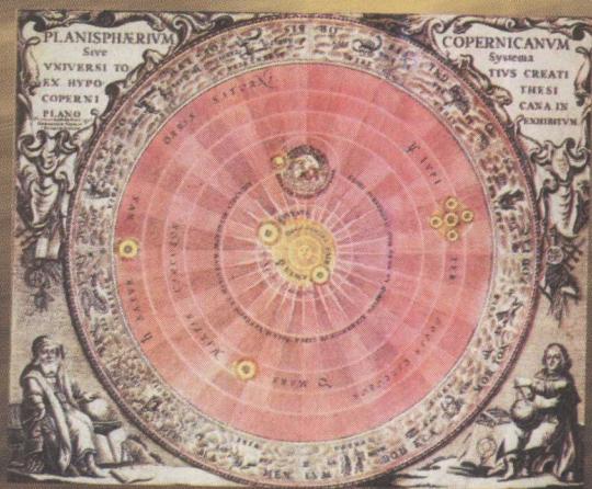
哥白尼《天体运行论》中的“日心说”示意图，他是把行星依次放在它们适当位置上的第一人
