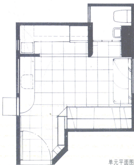
单元平面图
