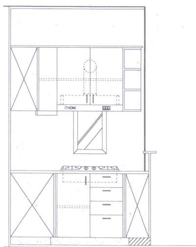
橱柜立面图 2
