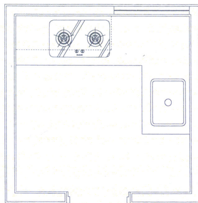
厨房平面图
