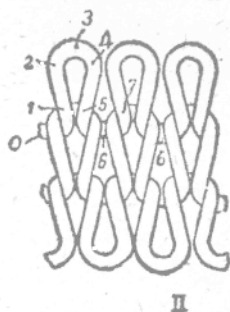
图 2 II—緯編針織物
