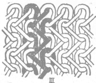
图 2 III—經編針織物
