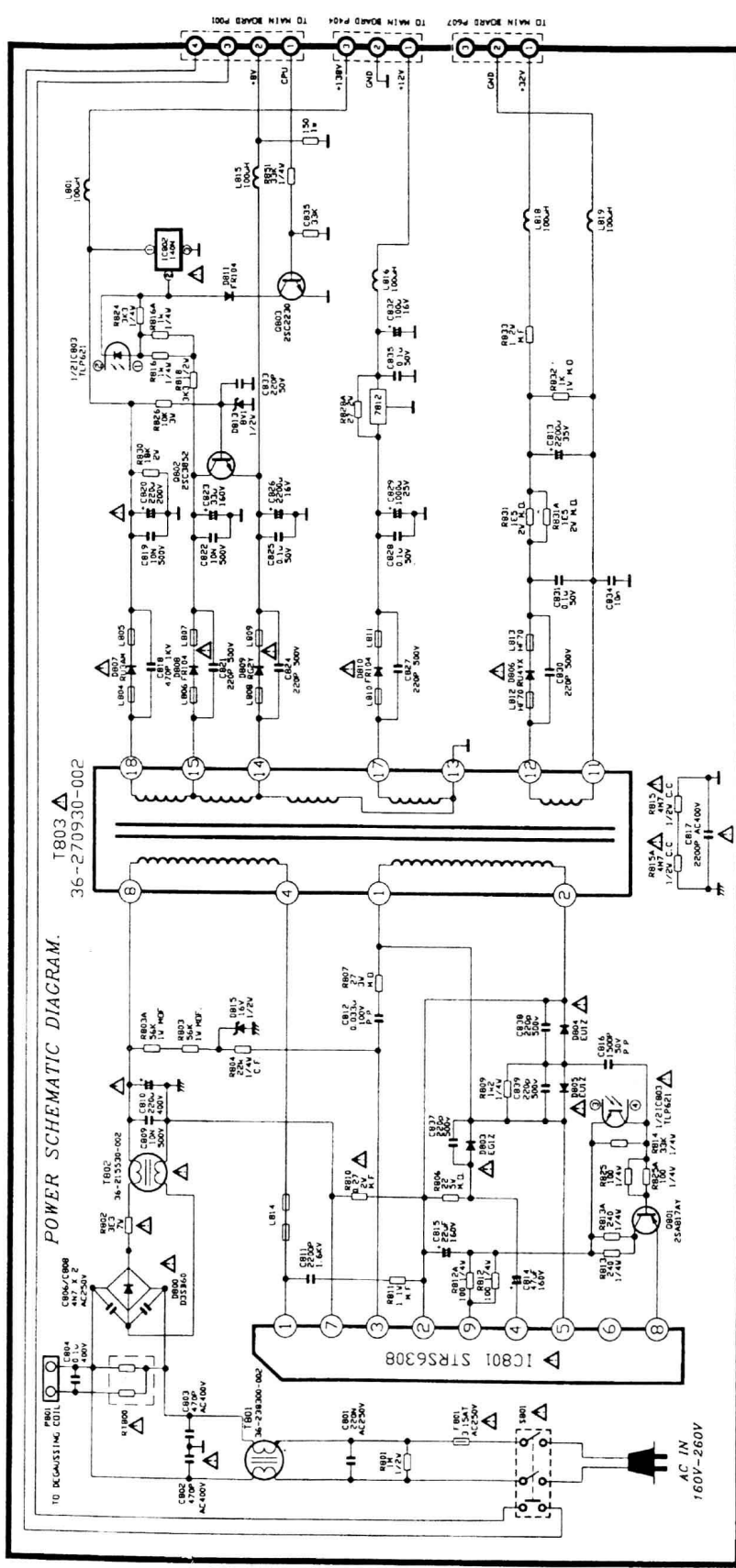
TCL-2568 电源及遥控电路板线路图
