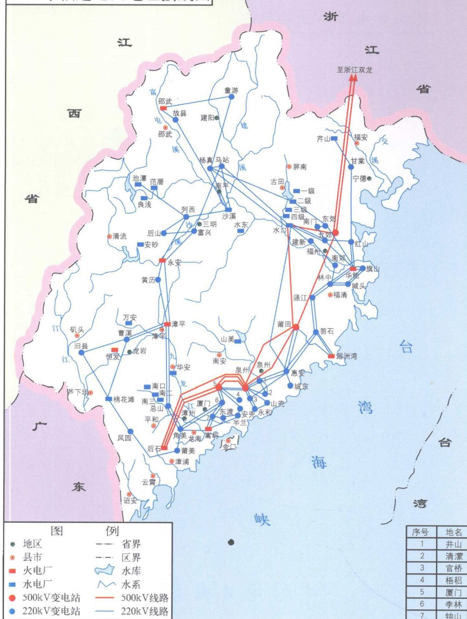
2002年福建电网地理接线图
