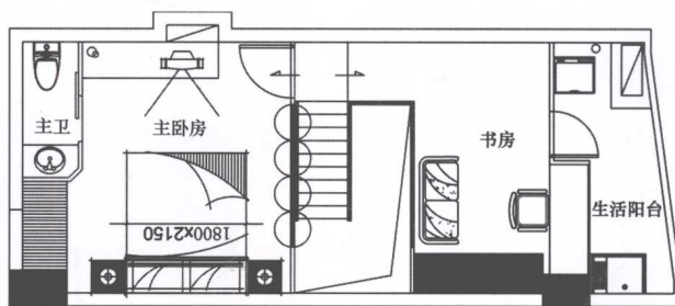
二层平面布置图
