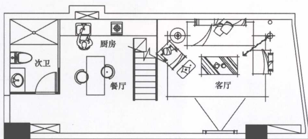
一层平面布置图
