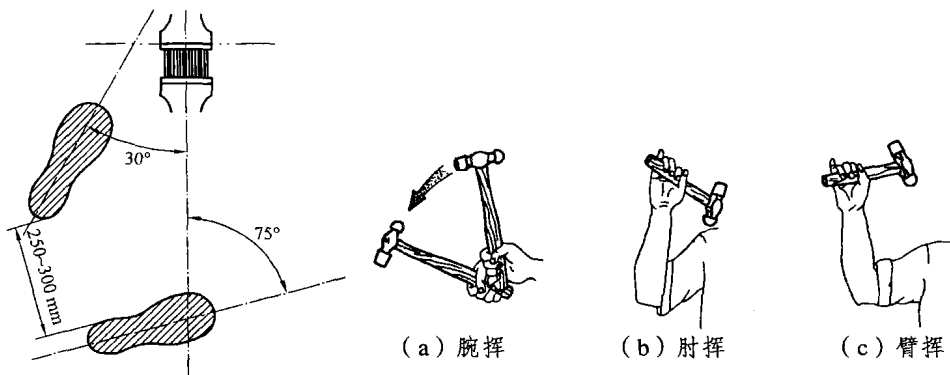
图 1.5 錾削工件时的站立位置
