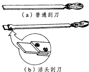
图 1.13 平面刮刀
