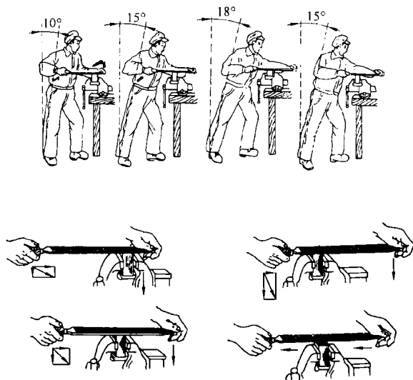
图 1.9 锉削姿势
