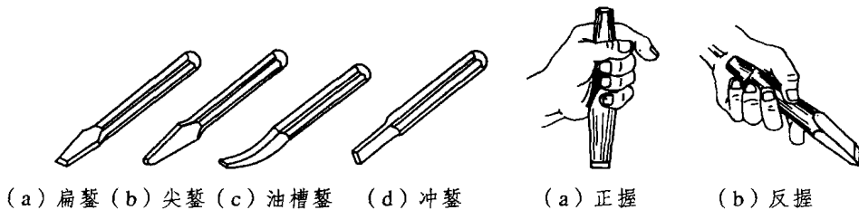
图 1.3 錾子
