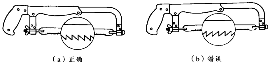
图 1.11 锯条的安装方法
