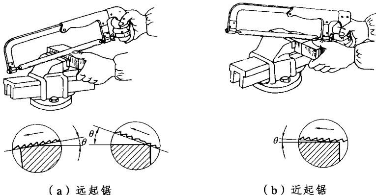
图 1.12 起锯
