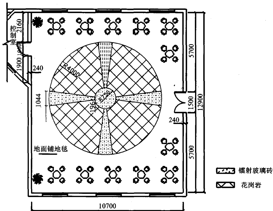
图 1—7 某舞厅地面铺贴示意图
