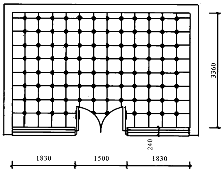
图 1—2 某店铺地面铺贴示意图
