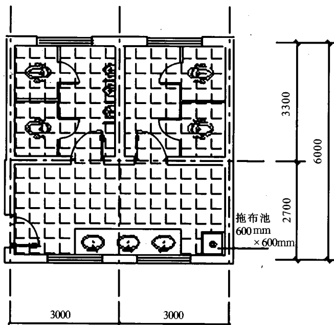
图 1—5 某建筑卫生间地面铺贴示意图
