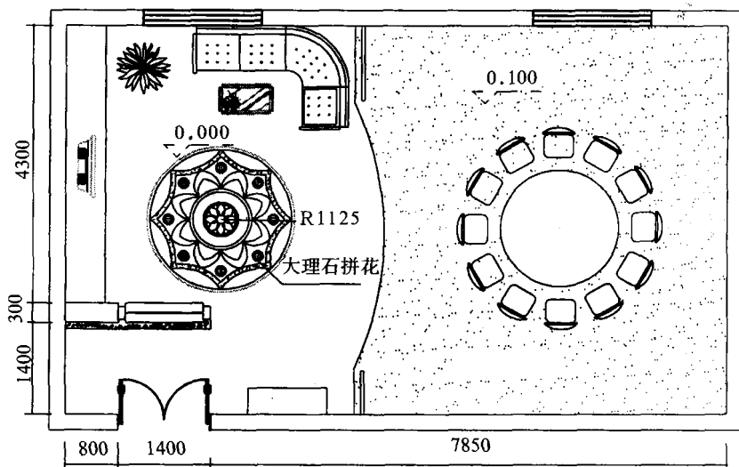
图 1—6 某餐厅地面铺贴示意图
