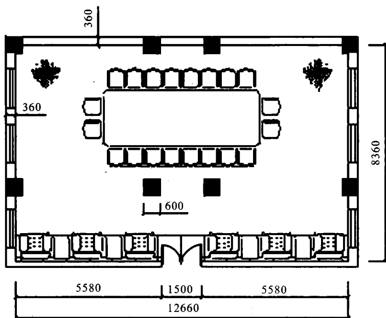
图 1—1 某会议室地面铺贴示意图
