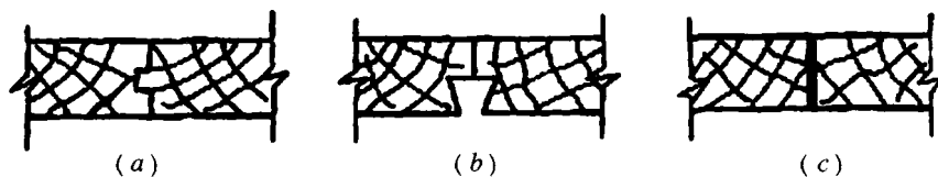
图 1—4 拼花木地板接缝
