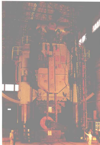
我国已形成门类比较齐全的机械制造体系。图为安装在上海重型机器厂的我国自行设计制造的12000吨压力的自由锻造水压机。
