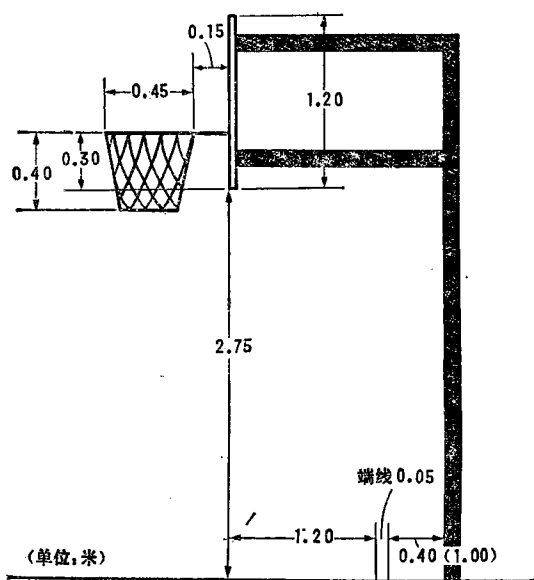
图三 篮架和球篮
