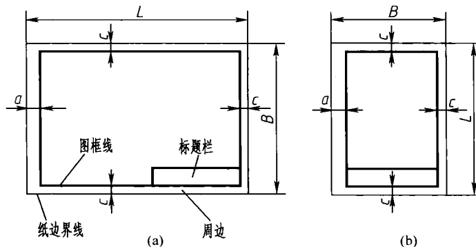
图 1-3 留有装订边的图框格式
