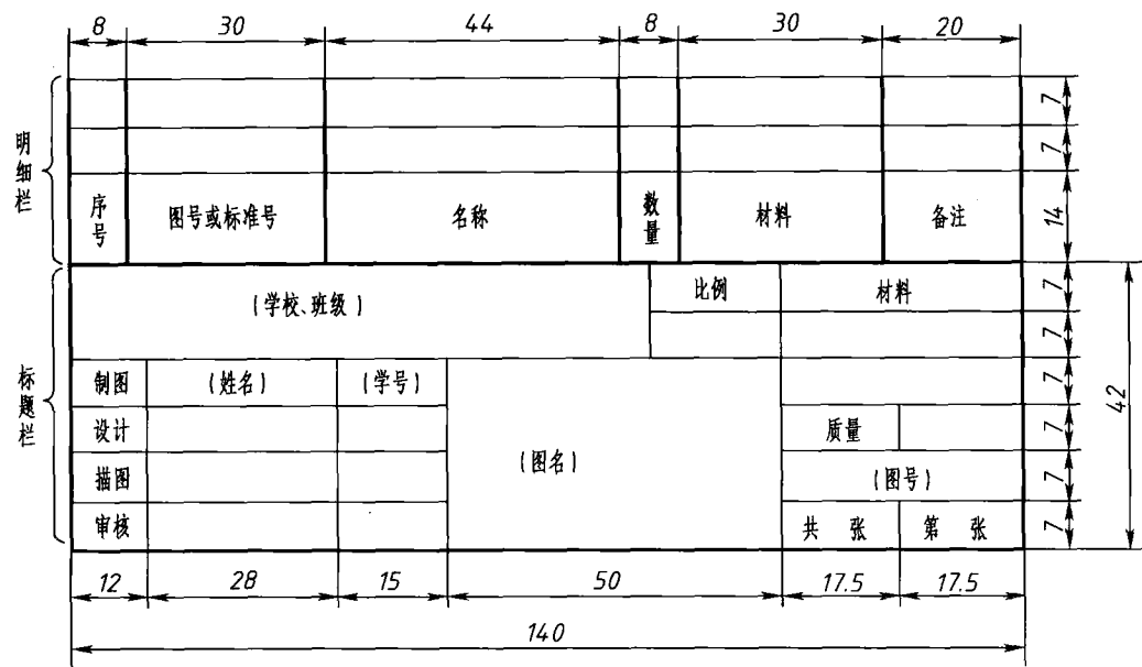
图 1-4 制图作业用标题栏及明细栏的格式
