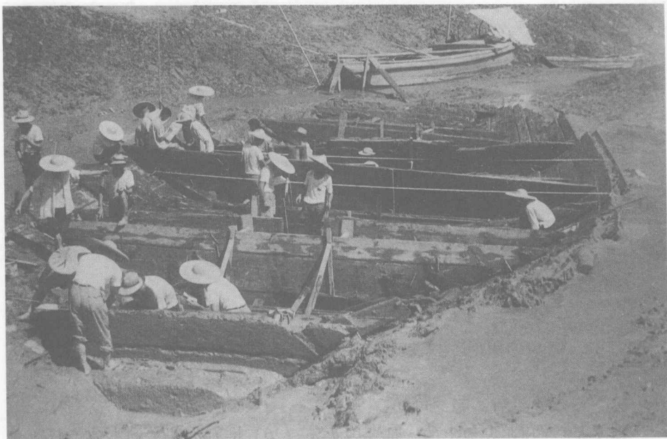
图 30 泉州市后渚港出土的古船遗骸
