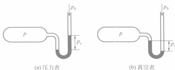
图 1-4 测压原理
