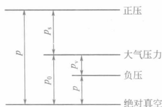
图 1-5 绝对压力与表压力、真空度的关系
