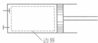
图 1-3 活塞式压缩机的 汽缸活塞系统
