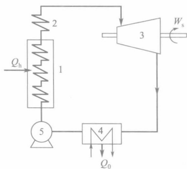
图 1-1 蒸汽动力循环
