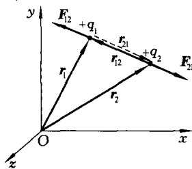
图 11.2 库仑定律
