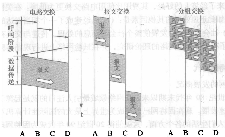
图 1-4 三种交换的比较 (P 1 ~P 4 表示 4 个分组)
