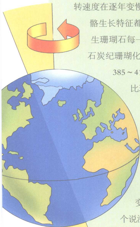
地球自转示意图
