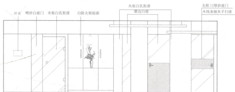
■ 客厅立面图
