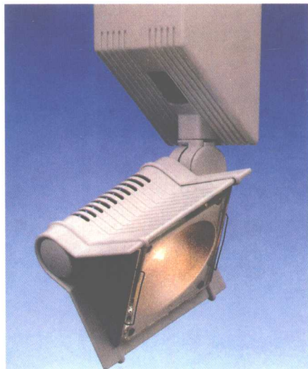
设计师：康兰设计小组，康克设计小组 照明设备 铸铝，钢杆 生产商：康克照明，英国
