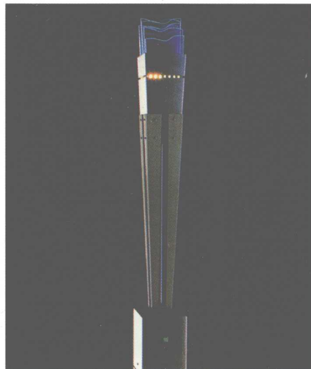
设计师：詹姆斯·伊万森 台灯 木、亚光处理铝 高：40厘米，底座：30厘米见方 生产商：曼菲思，意大利
