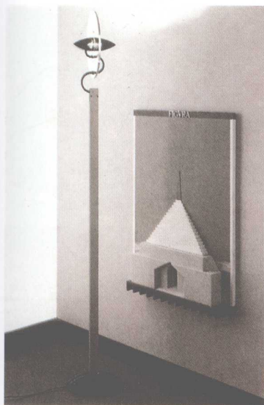
设计师：卡罗·伏科里尼 落地灯 有灰和黑色 铝，玻璃灯罩 最大300瓦卤素灯 高：201厘米，宽：35厘米 生产商：阿特梅德，意大利
