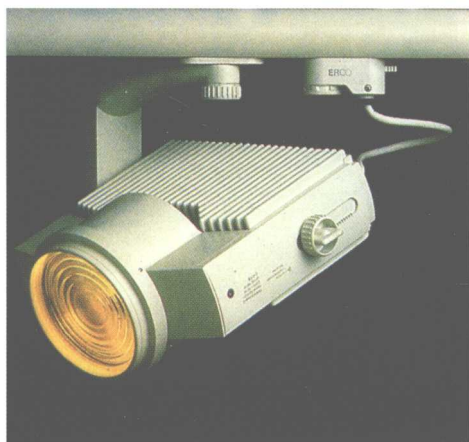
设计师：马里奥·贝里尼 灯 低压探照灯 可换50瓦、75瓦、100瓦的灯泡 直径：12.5厘米，宽：27.8厘米，长：25.9厘米，宽：21.6厘米 生产商：埃克，德国
