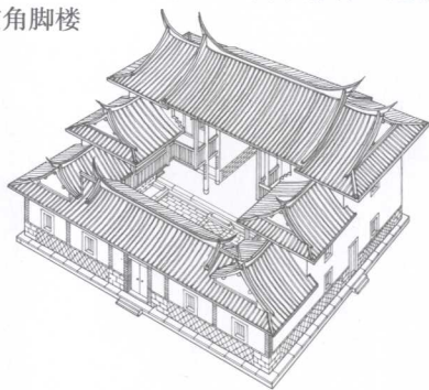
图 2-1-9 五间起虎头厝鸟瞰图
