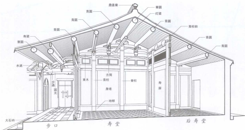
图 1-3-5 泉州市金鱼巷 114 号大厅剖视图
