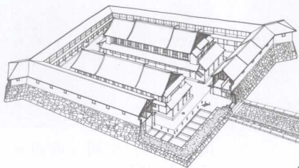
图 2-1-14 德化县三班镇硕杰村大兴堡剖视图
