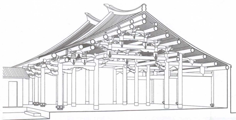
图 1-3-4 插梁坐梁式构架
