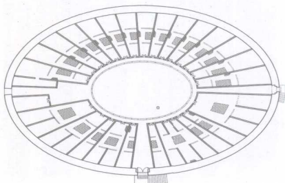
图 2-1-25 华安县沙建镇岱山村齐云楼平面图
