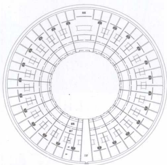
图 2-1-24 漳州市平和县九峰乡黄田村龙见楼平面图
