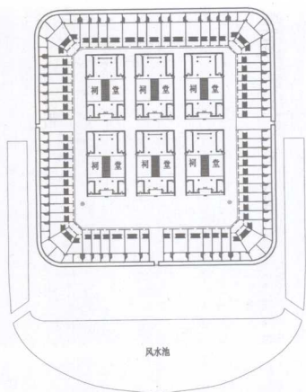
图 2-1-21 平和县霞寨乡西爽楼平面图
