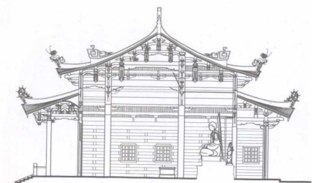
图 2-3-10 厦门南普陀寺 大雄宝殿剖面图
