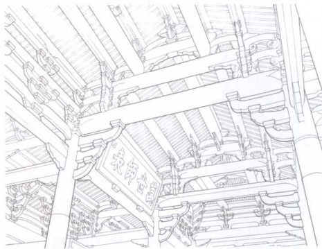
图 2-4-3 泉州文庙大成殿纵架
