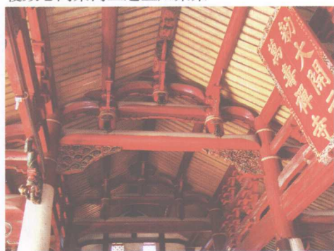
图 2-3-2 泉州开元寺天王殿梁架
