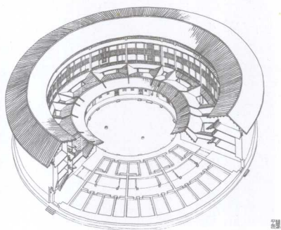
图 2-1-22 华安县仙都镇大地村二宜楼剖视图
